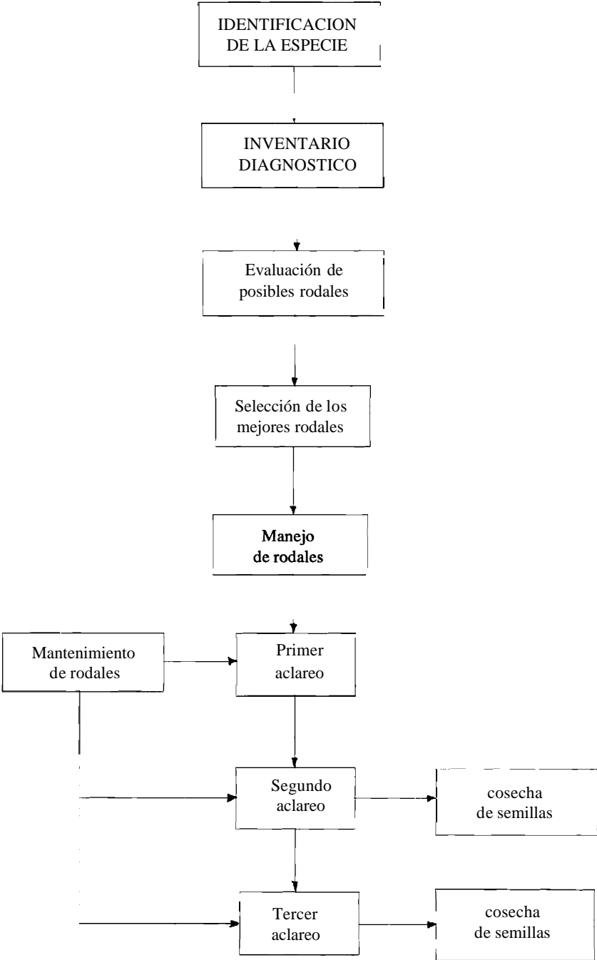
Figura 6. Proceso para establecer y manejar un rodal semillero.
