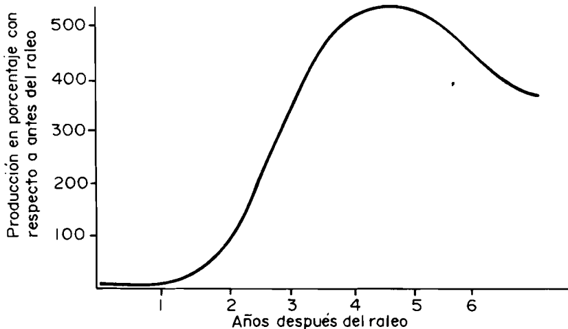
Figura 15. Comportamiento de la producción de semillas después de establecido el rodal semillero de Pinus taeda , (Zobel y Talbert, 1988).
