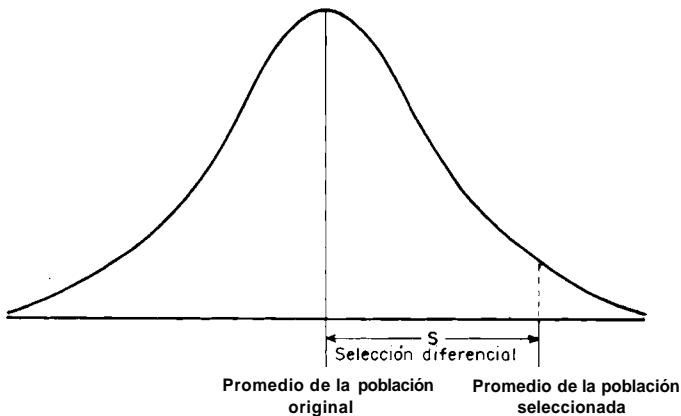
Figura 2. La selección diferencial es la diferencia entre la media de la población original y la media de la población seleccionada.
