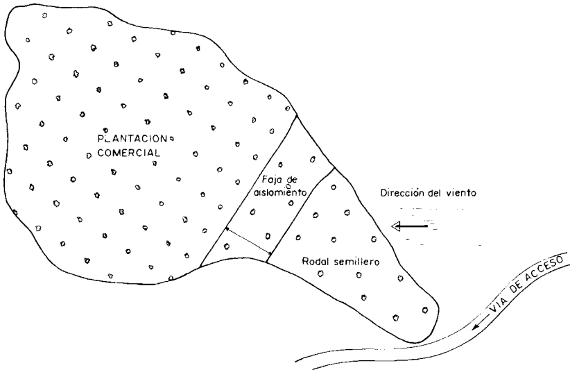
Figura 11. Si la plantación es grande, seleccionar para rodal semillero la parte con mejor acceso, mejor crecimiento y con menor riesgo de contaminación de polen de la misma plantación.
