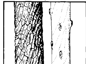
Figura 7. Rasgos morfológicos más comunes en C. lusitánica : A. rectitud del fuste, R. grosor de ramos, C. ángulo de insición ramos-fuste, D. bifurcación y E. grano en espiral. (R. Quirós).
