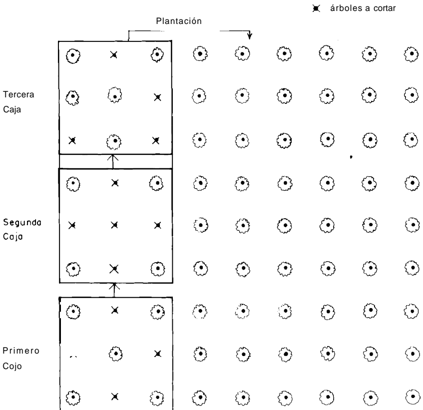
Figura 13. Sistema de caja (grupo) de nueve árboles para facilitar la ejecución de un aclareo de 50%.
