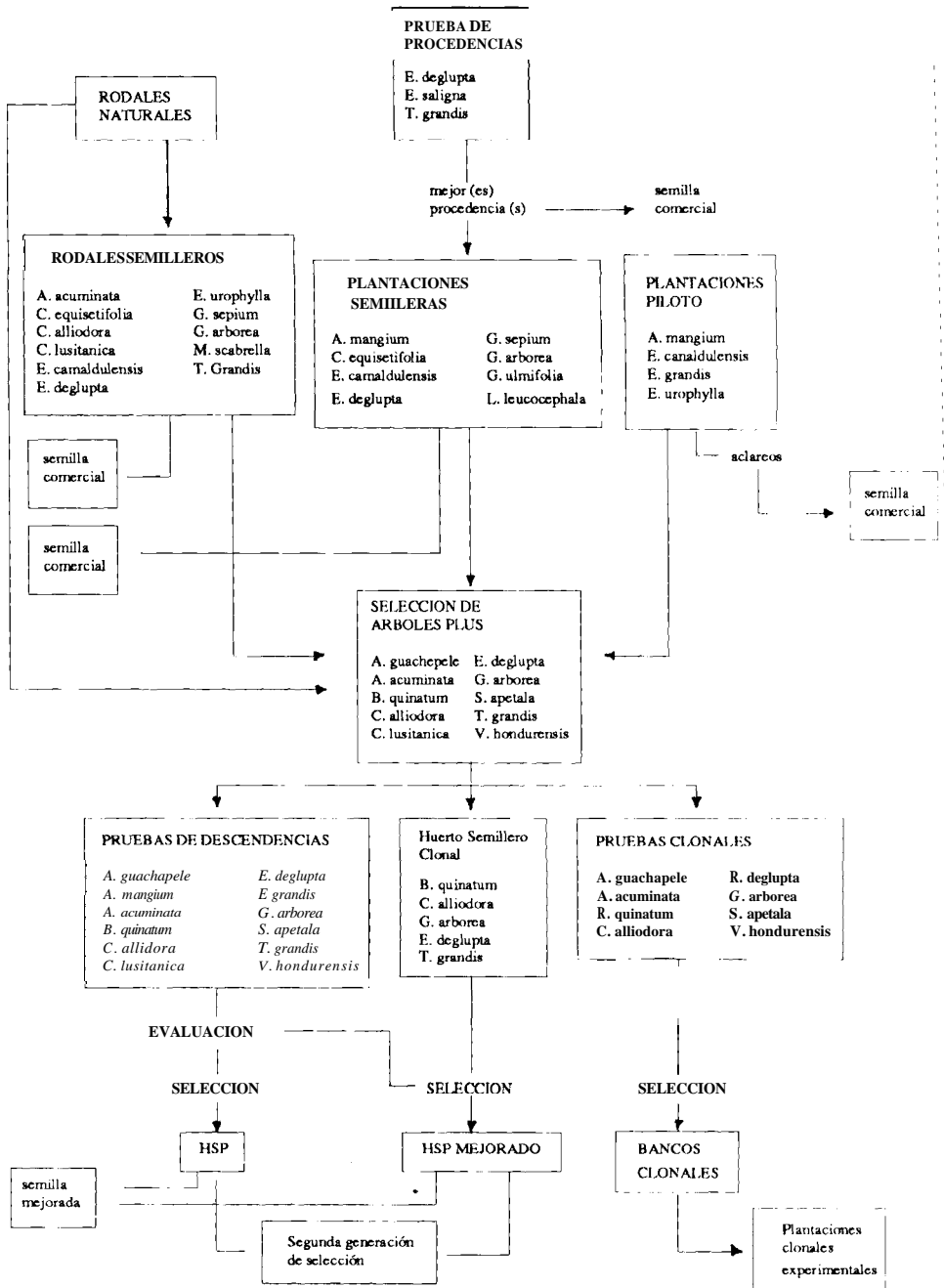
Figura 3. Una estrategia de mejoramiento genético forestal en algunas especies prioritarias de América Central (F. Mesén)
