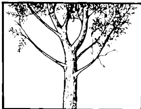
Figura 7. Rasgos morfológicos más comunes en C. lusitánica : A. rectitud del fuste, R. grosor de ramos, C. ángulo de insición ramos-fuste, D. bifurcación y E. grano en espiral. (R. Quirós).
