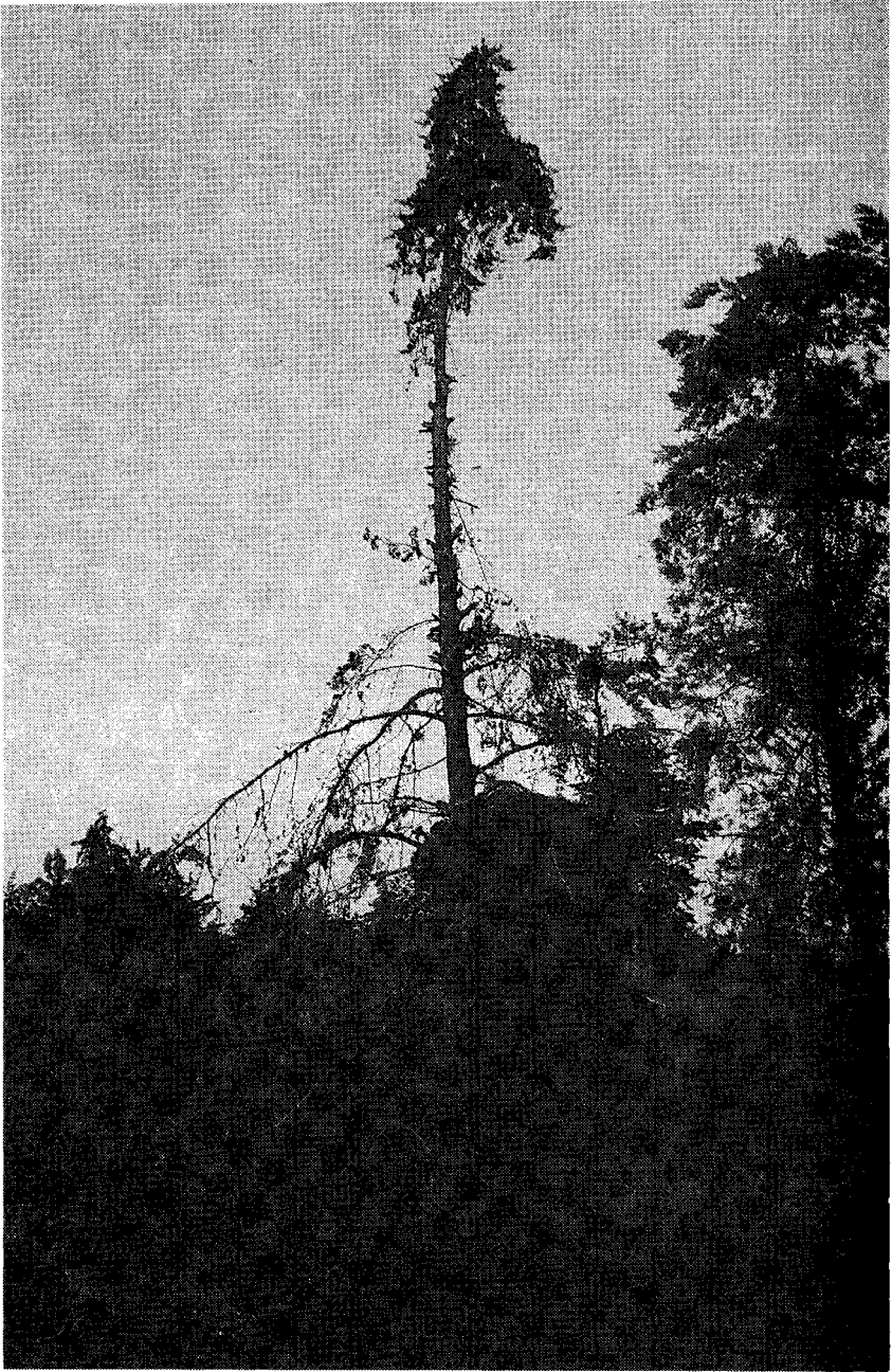
Figura 16. Para cosechar las semillas no destruya la copa del árbol. (Foto: R. Salazar).
