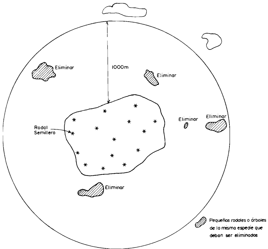
Figura 10. Es conveniente eliminar fuentes de contaminación en un radio de 1000m alrededor del rodal semillero.
