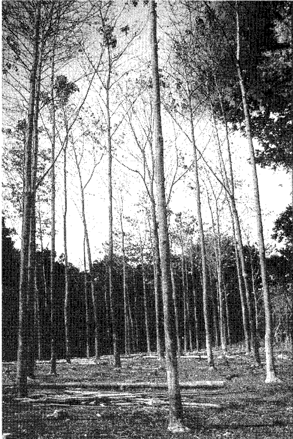
Figura 4. Rodal semillero de Gmelina arborea en Hojancha, Costa Rica. (Foto: D. Boshier).
