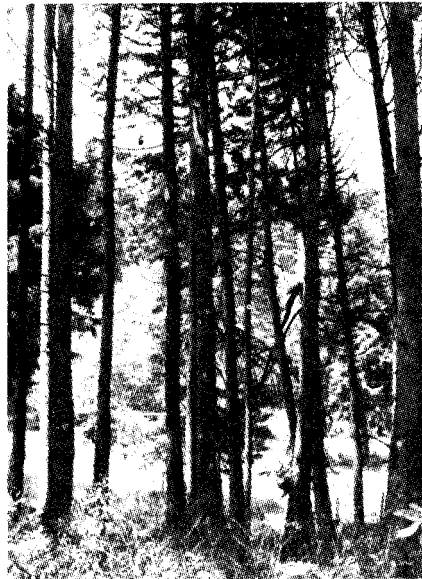
Figura 8. Rodal natural de Cupressus lusitanica bajo manejo para rodal semillero en Guatemala.
