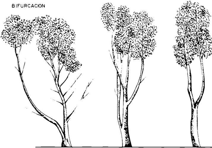
Figura 9. Algunas características morfológicas que predominan en Gmelinaarhorea .
